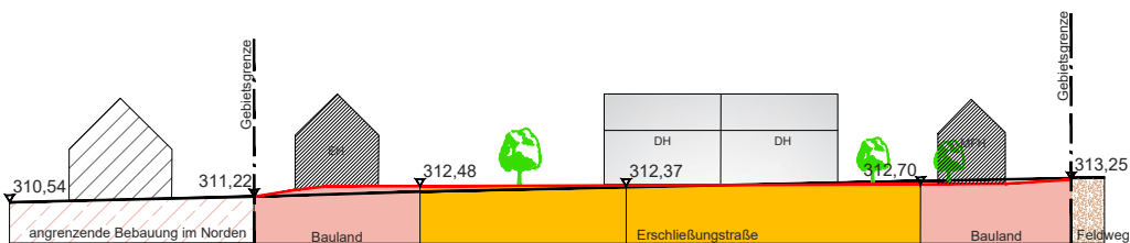
SCHEMA-SCHNITT - ACHSE D - BLICK RICHTUNG OST
