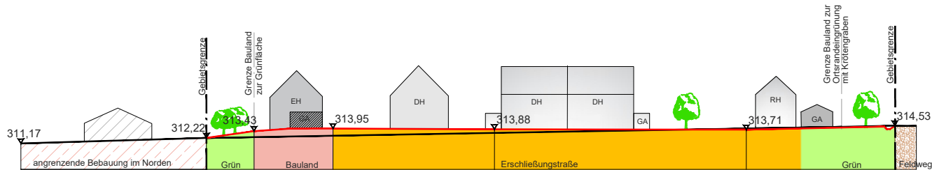
SCHEMA-SCHNITT - ACHSE A - BLICK RICHTUNG OST
